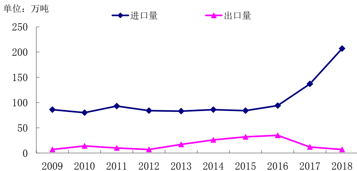
图 30 箱纸板 2009~2018 年进口量及出口量
