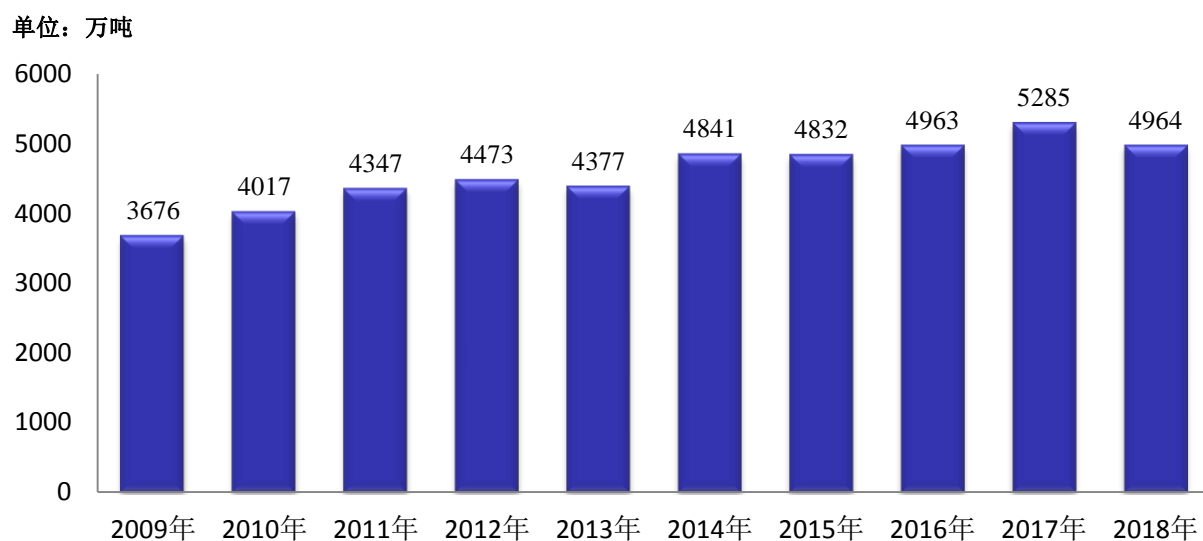
图 18 2009~2018 年全国废纸回收总量
